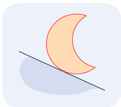
Через эту точку фигуры проходит лишь одна опорная прямая
