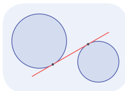
Общая внутренняя касательная
