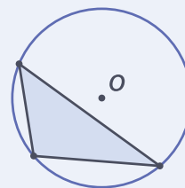
окружность тупоугольного треугольника
