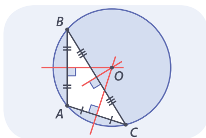
Серединные перпендикуляры к сторонам любого треугольника пересекаются в одной точке
