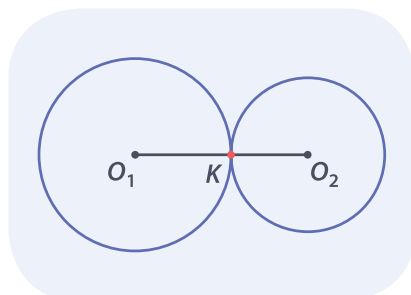
Внешнее касание окружностей
